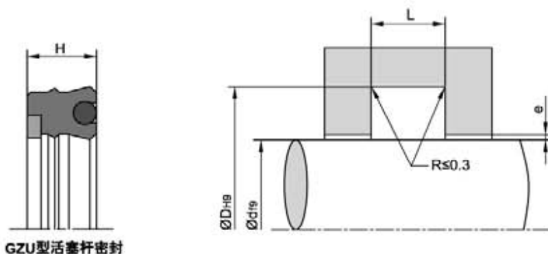
GZU型活塞杆密封
