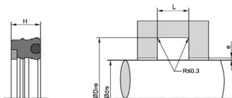
GZU型活塞杆密封
