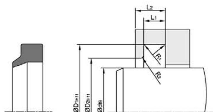
GA5型防尘圈
