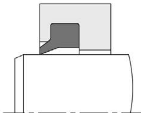
GA5型防尘圈
